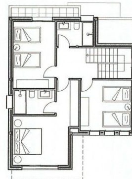
PLANTA ALTA
