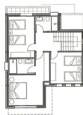
PLANTA ALTA
